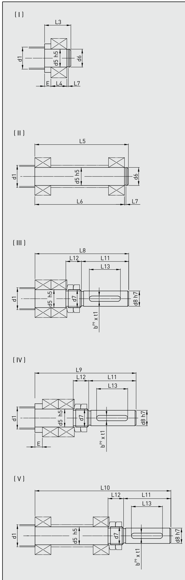
Fig. 3.7: Configurazioni dei terminali dell'albero
