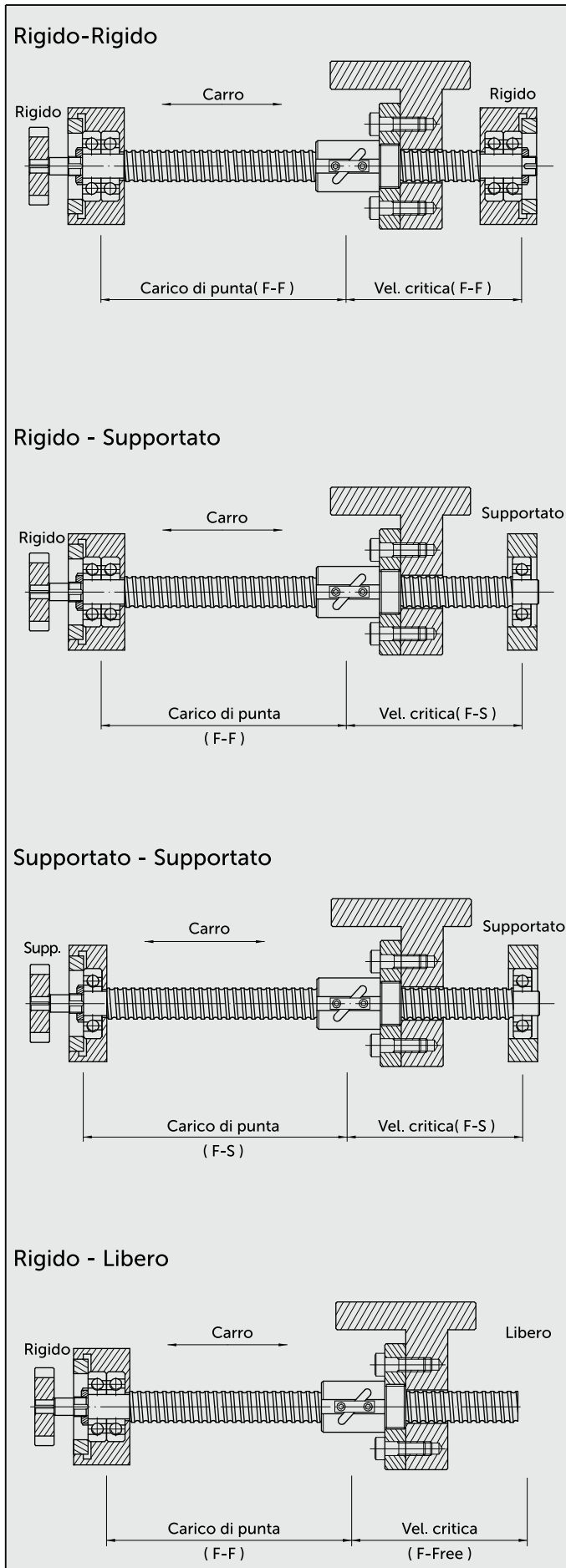
Fig. 3.6: Metodi di montaggio consigliati per i punti di appoggio dei terminali delle viti a ricircolo di sfere
